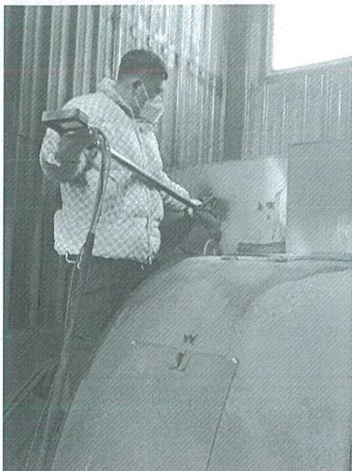
附图 1 锅炉废气采样图
