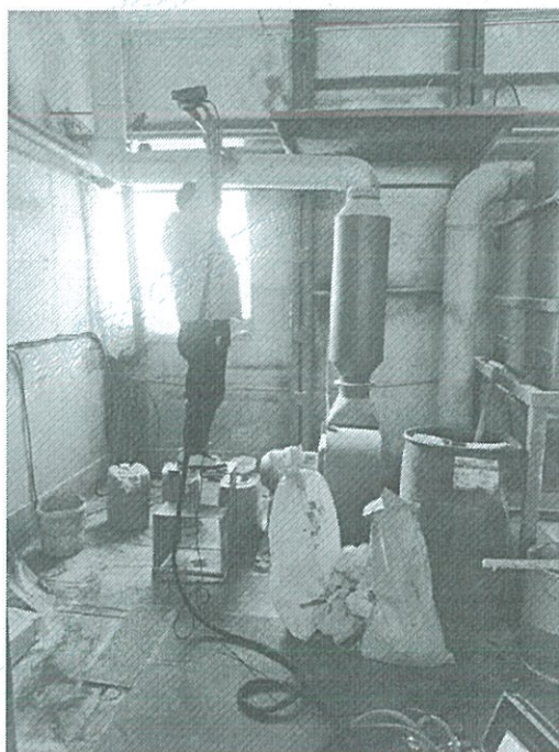
附图 2 有组织废气采样图
